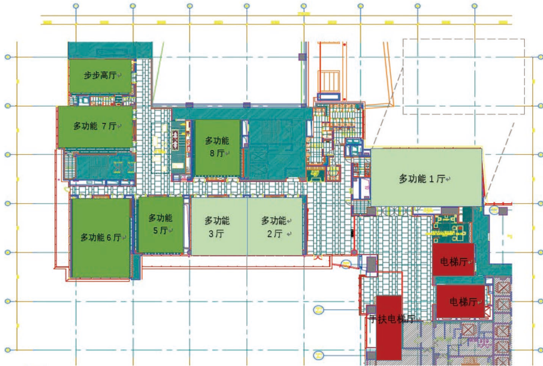
五楼 平面布局图
